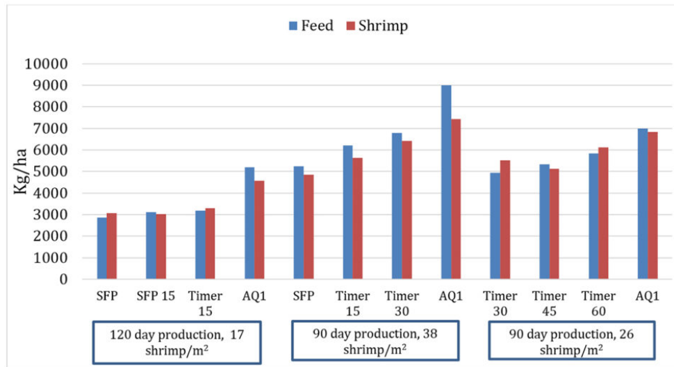
Fig. 2: Resumen de tres años del alimento total utilizado y la biomasa final del camarón.
